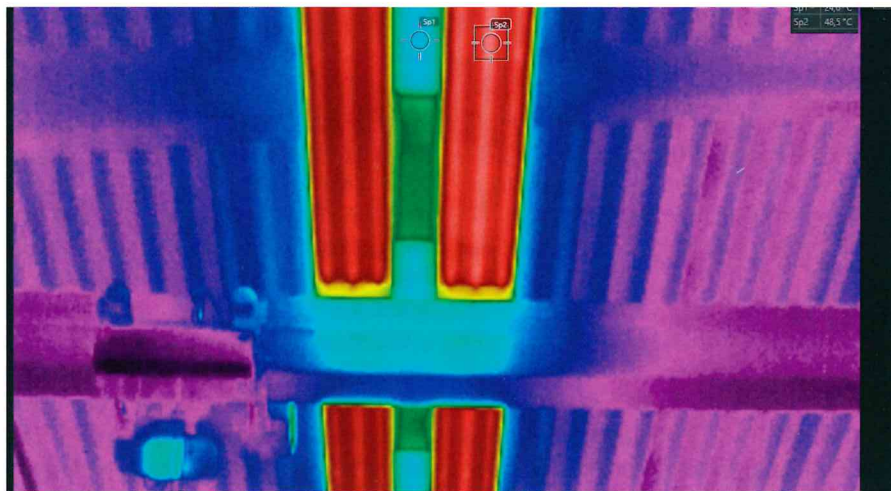
Die Thermografie-Aufnahme zeigt die thermische Entkoppelung der Strahlfläche von den LED-Leuchten.
