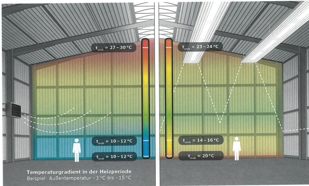
Die Temperaturschichtung in einer Halle bei Luftheizung (links) und Deckenstahlheizung (rechts). ( t_{amb} = ambient operating temperature, zu Deutsch: Betriebsumgebungstemperatur).
